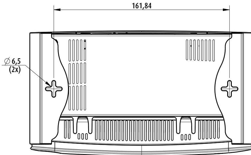
Obrázek 4-1: Montážní otvory
