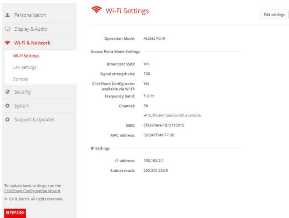
Obrázek 6-17: Nastavení WiFi
