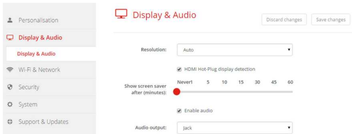
Obrázek 6-15: Nastavení displeje
