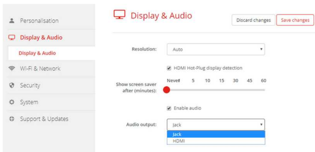
Obrázek 6-16: Nastavení zvuku
