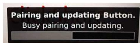
Obrázek 5-2: Párovací zpráva
