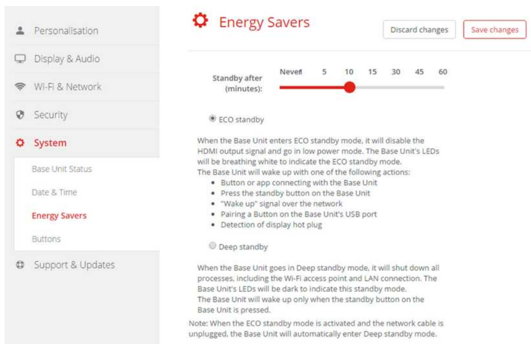
Obrázek 6-42: Spořiče energie
