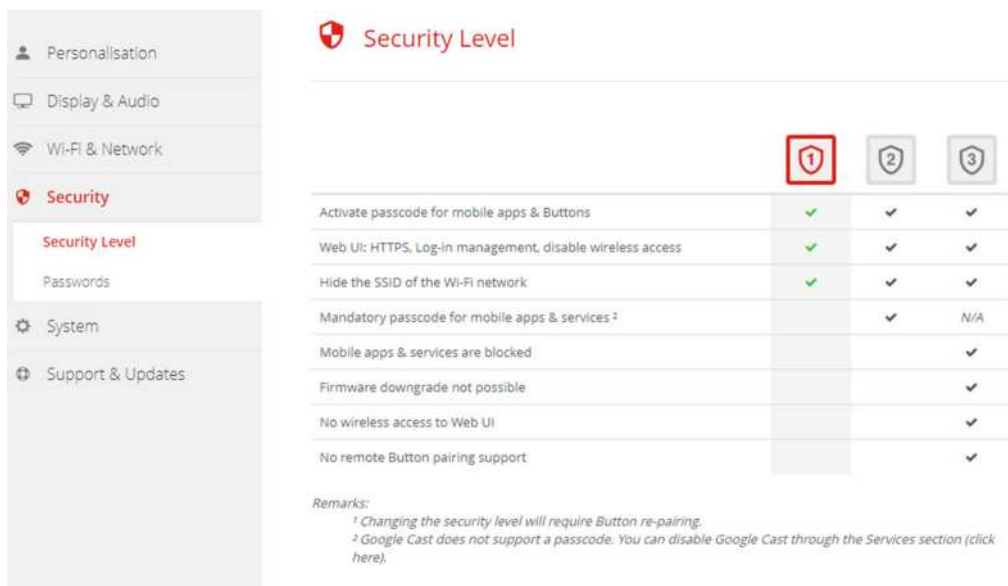
Obrázek 6-31: Úrovně zabezpečení
