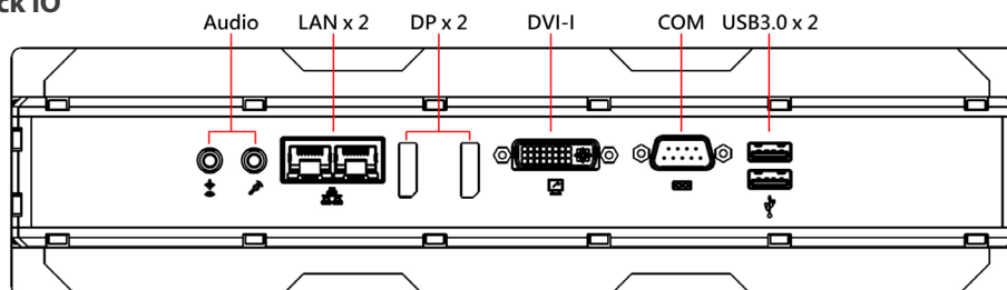
Back IO
